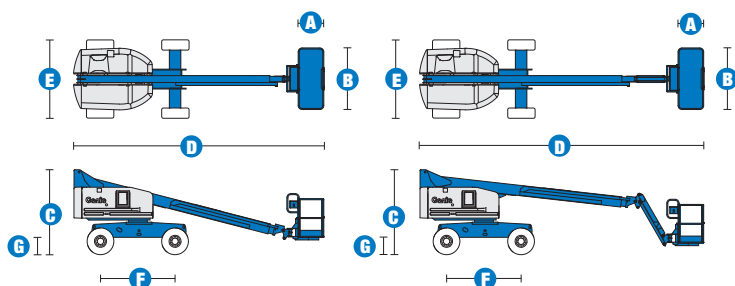
DIAGRAMMA DI LAVORO S™-40
