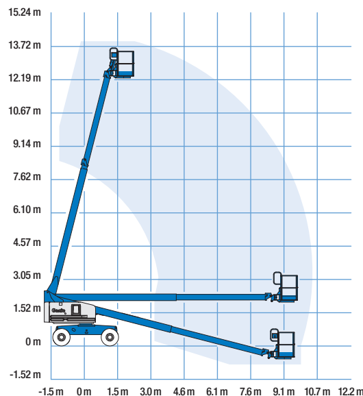
DIAGRAMMA DI LAVORO S™-40
