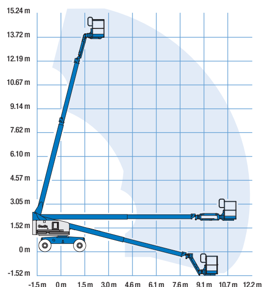
DIAGRAMMA DI LAVORO S™-45
